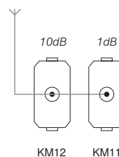
последовательное соединение throughpass connection
