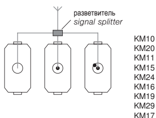
соединение «звездочка» star connection
