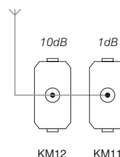
преходно свързване throughpass connection
