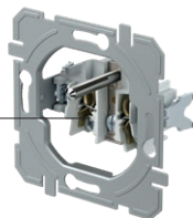
винтови контакти screw contacts
