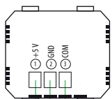
външно устройство exterior unit
