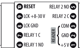
вградено релейно устройство interior relay unit
