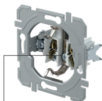
csavaros érintkezők screw contacts
