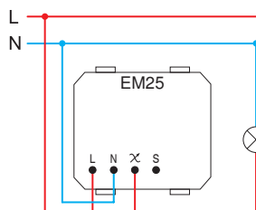
(2) három vezetékű csatlakozás three-wire connection
