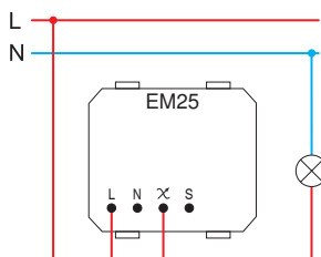
(1) két vezetékű csatlakozás two-wire connection
