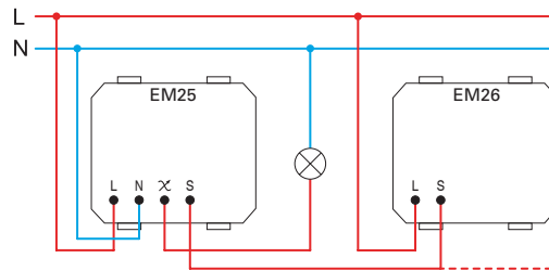
(2) trožična vezava three-wire connection
