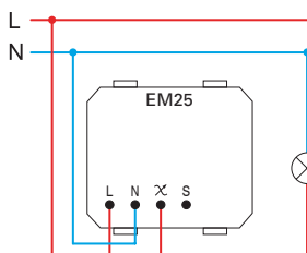
(2) trožična vezava three-wire connection
