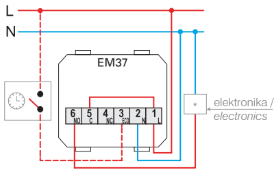
obtočna črpalka, gorilnik (direktna priključitev), termoelektrični pogon / circulation pump, burner (direct connection) thermoelectric drive
